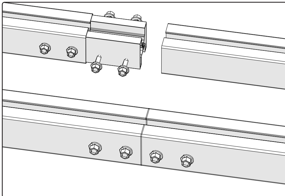
Abb. 5 Montageschienen verbinden
