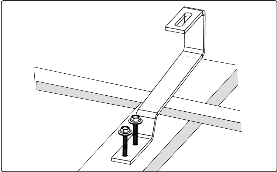
Abb. 3 Dachhaken montieren
