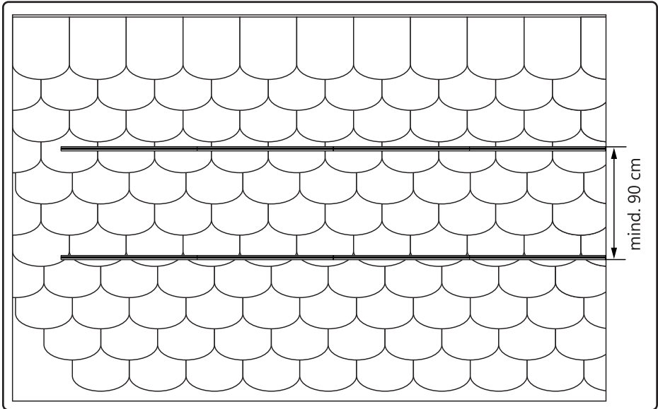
Abb. 2 Beispielhaftes Anzeichnen des Schienenabstands
