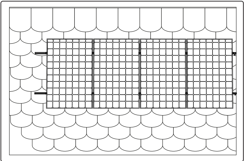
Abb. 10 Fertig montierte Solarmodule
