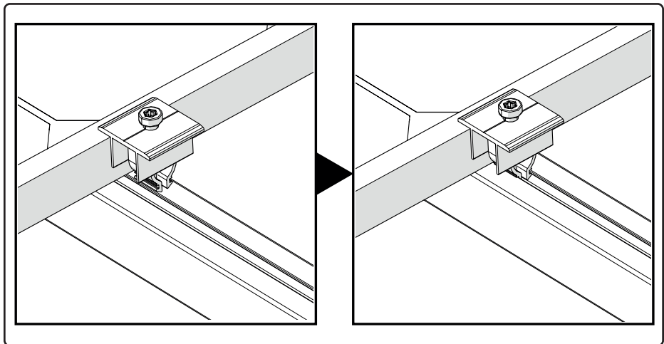
Abb. 7 Modulmittelklemmen einklicken
