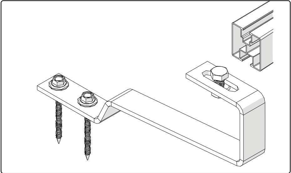
Abb. 4 Montageschiene in Dachhaken einführen
