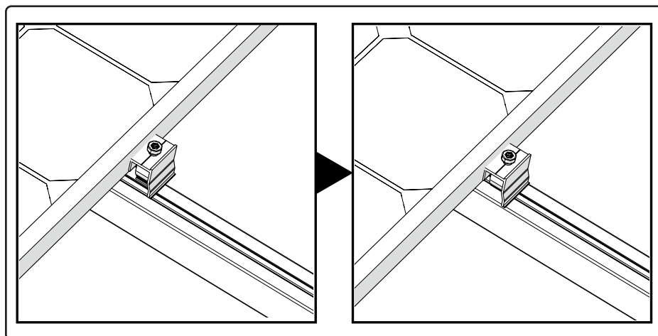
Abb. 8 Modulendklemmen einklicken
