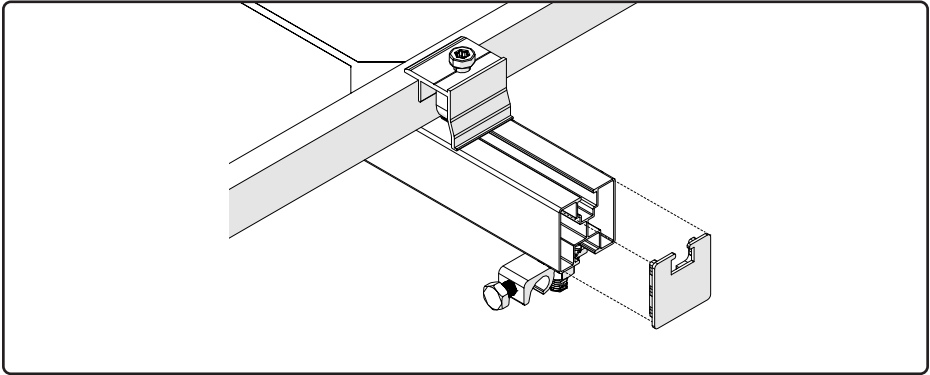
Abb. 9 Erdungsklemme und Gummiabdeckung montieren
