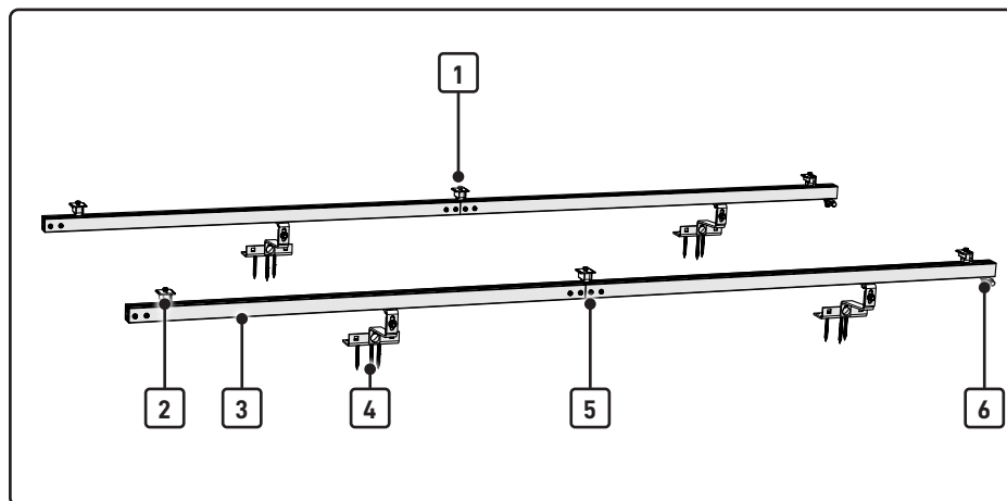
Abb.1 Montageset
