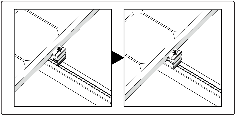
Abb. 8 Modulendklemmen einklicken
