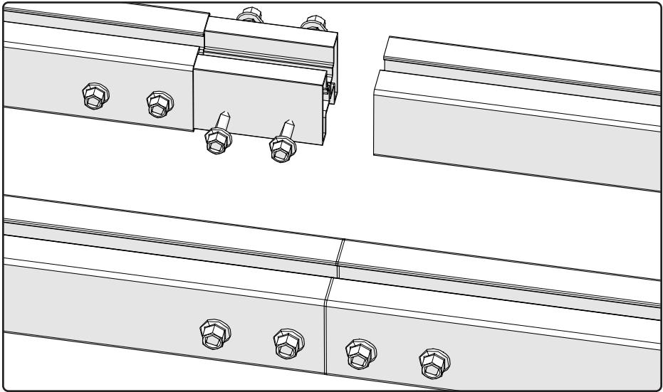
Abb. 6 Montageschienen verbinden
