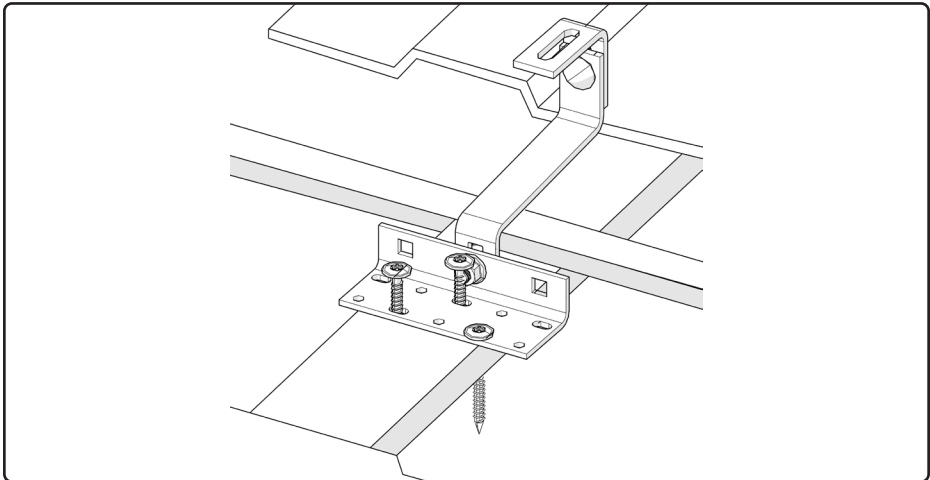
Abb. 3 Dachhaken montieren
