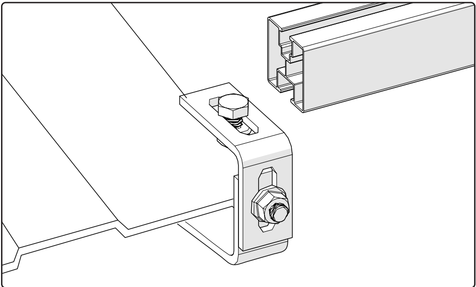
Abb. 5 Schiene in Dachhaken einführen
