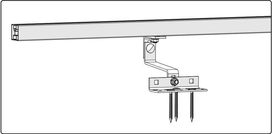
Abb. 4 Montageschienen
